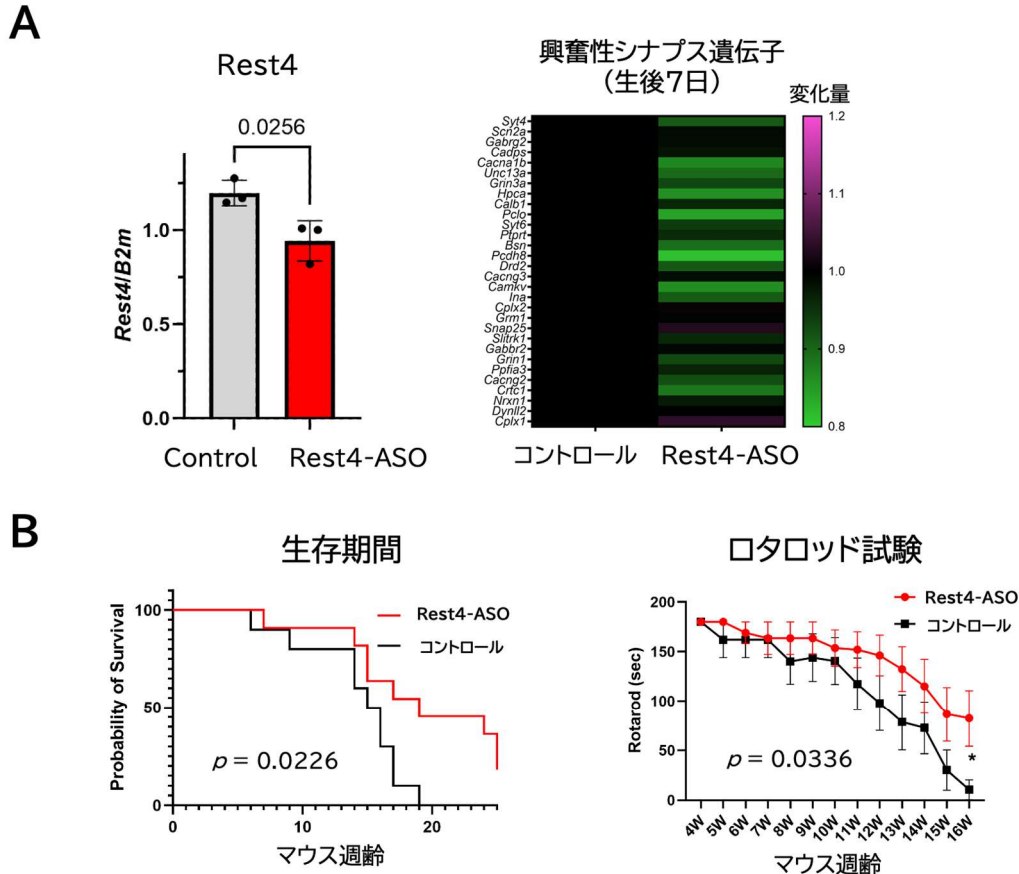
図5. 超早期に興奮性シナプスの遺伝子発現を低下させることで、SBMAマウスの生存期間や運動機能が改善する (A) Rest4-ASOによる興奮性シナプス遺伝子の低下 (生後1日に投与) (B) Rest4-ASOはマウスの生存期間を延長し、運動機能を改善する
