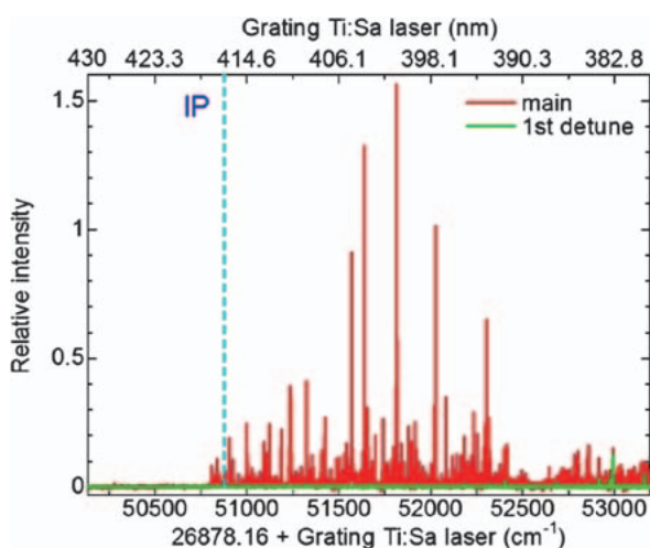
図3 Th イオン化ポテンシャル (IP) 近傍の共鳴スペクトル
